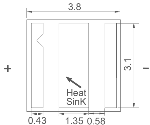
Fig.1-2 Bottom view 背面视图
