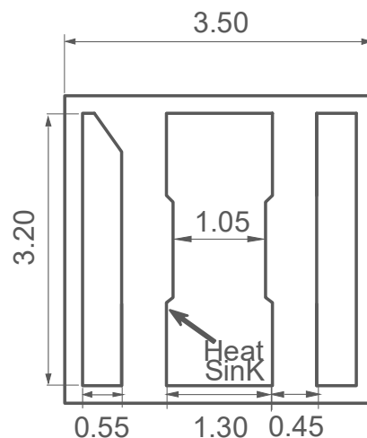
Fig.1-2 Bottom view 背面视图
