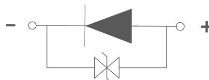
Fig.1-4 Polarity 极性
