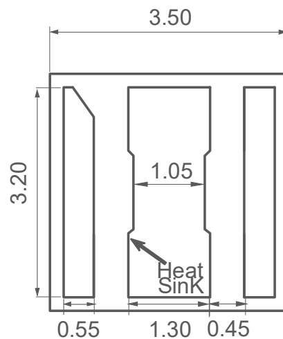
Fig.1-2 Bottom view 背面视图
