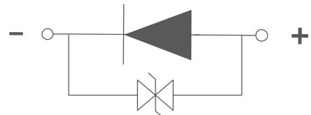
Fig.1-4 Polarity 极性
