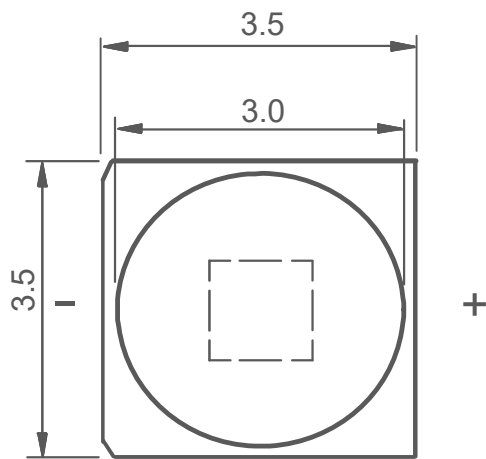
Fig.1-1 Top view 正面视图
