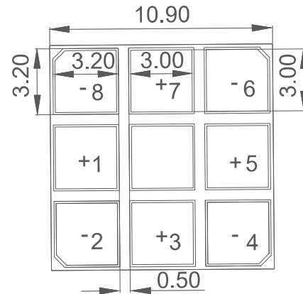
Fig.1-2 Bottom view 背面视图
