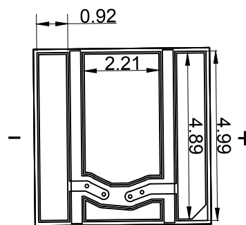
Fig.1- 2 Bottom view 背面视图
