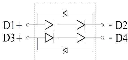
Fig.1-4 Polarity 极性
