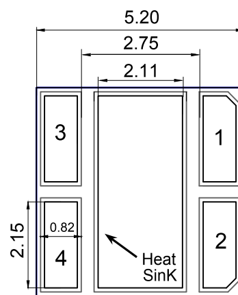
Fig.1-2 Bottom view 背面视图
