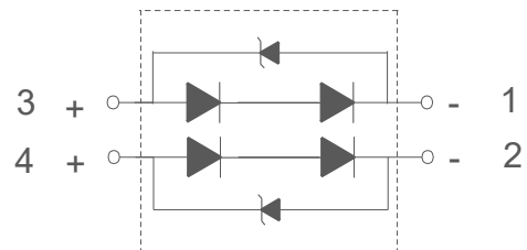
Fig.1-4 Polarity 极性
