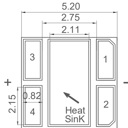
Fig.1-2 Bottom view 背面视图
